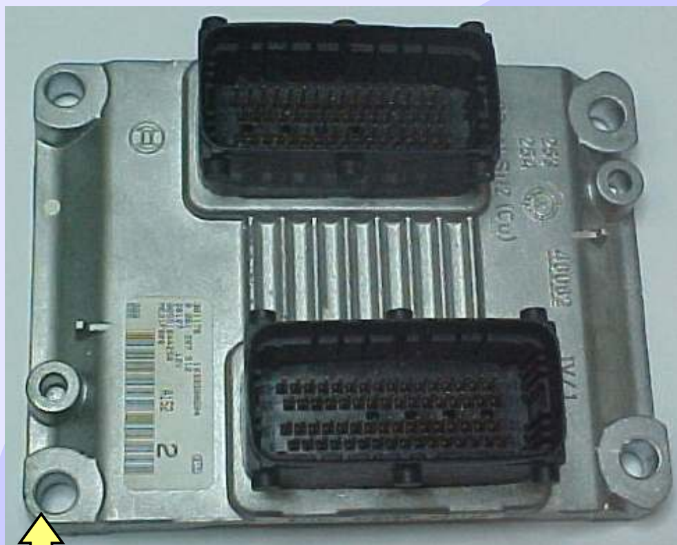
Central Híbrida Bosch ME 3.1 513 0261 207 513
