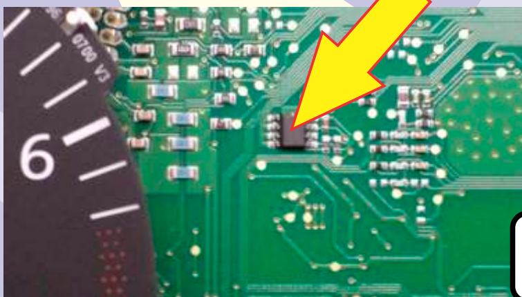
Localizando a memoria Soic 8 - 24C64
